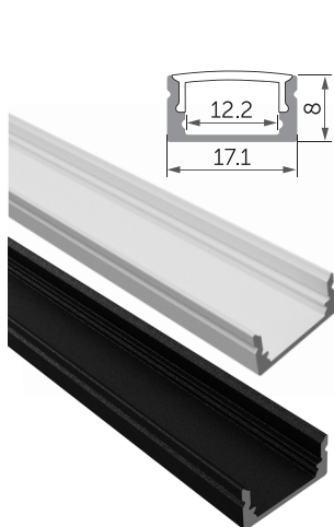
2M QLP ALUPROFIL 1 El.nr.: 3200895 - Hvit El.nr.: 3201061 - Sort
