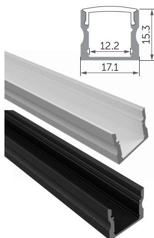
2M QLP ALUPROFIL 2 El.nr.: 3200896 - Hvit El.nr.: 3201062 - Sort
