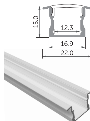
2M QLP ALUPROFIL 4 2meter aluprofil Hvit m/ flens H15mm x B23mm El.nr.: 3201063
