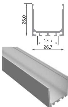
2M QLP ALUPROFIL 5 2meter aluprofil Hvit H26mm x B27mm El.nr.: 3201064
